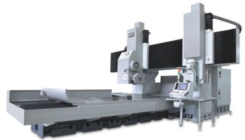
龍門磨床
